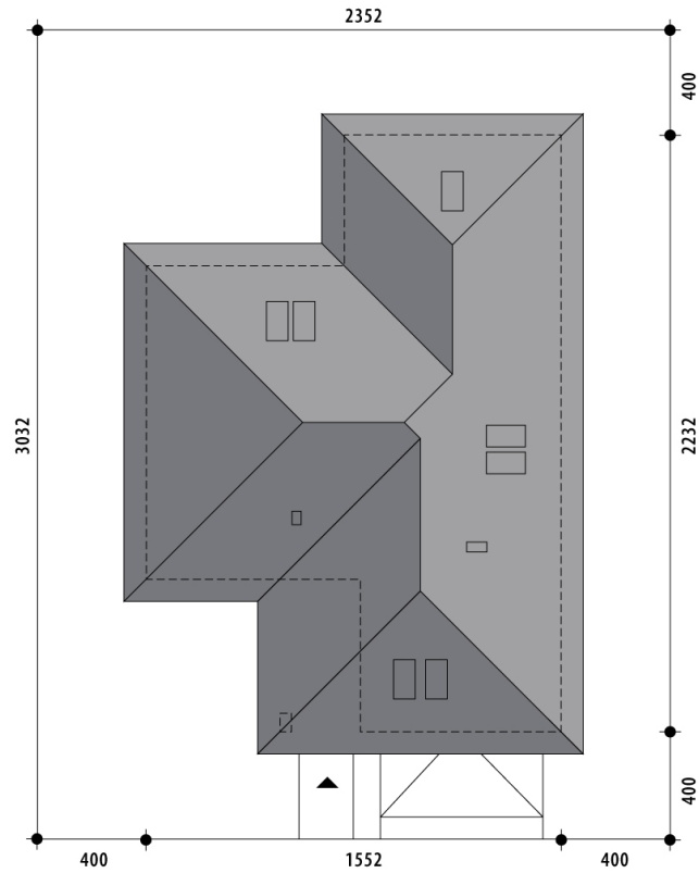
RZUT DZIAŁKI
