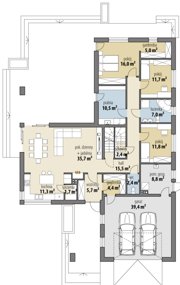
RZUT PARTER
