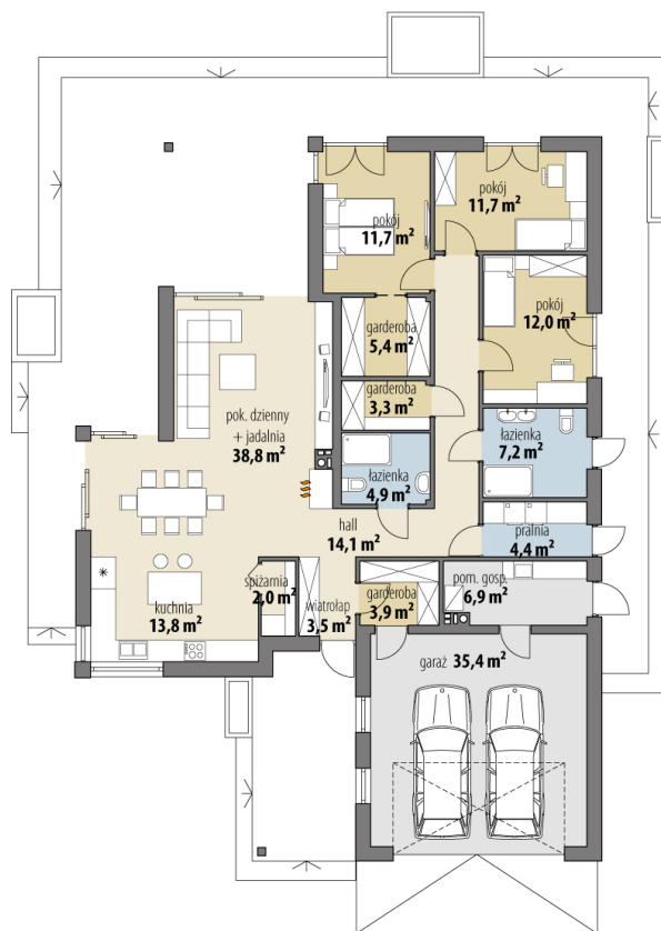
RZUT PARTER
